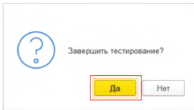
Рисунок 7. Завершение тестирования
